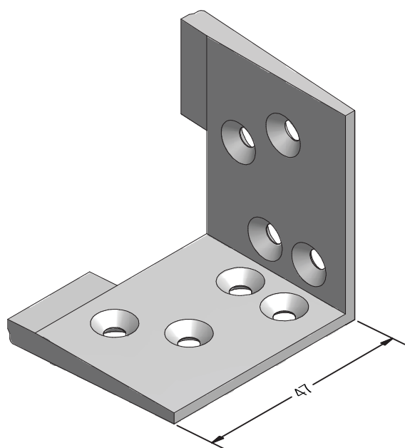
Монтажный уголок для горбылька BT 70 литой металлический
