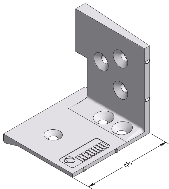
Монтажный уголок для створки Z 54 литой металлический
