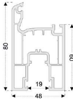
Sliding Door Sash Profile
