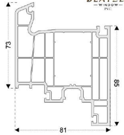
Inward Opening Door Profile
