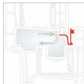
La creșterea presiunii vântului sistemul REHAU AirComfort se închide automat, pe baza principiului lui Bernoulli.
