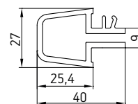
035 Соединитель-усилитель
