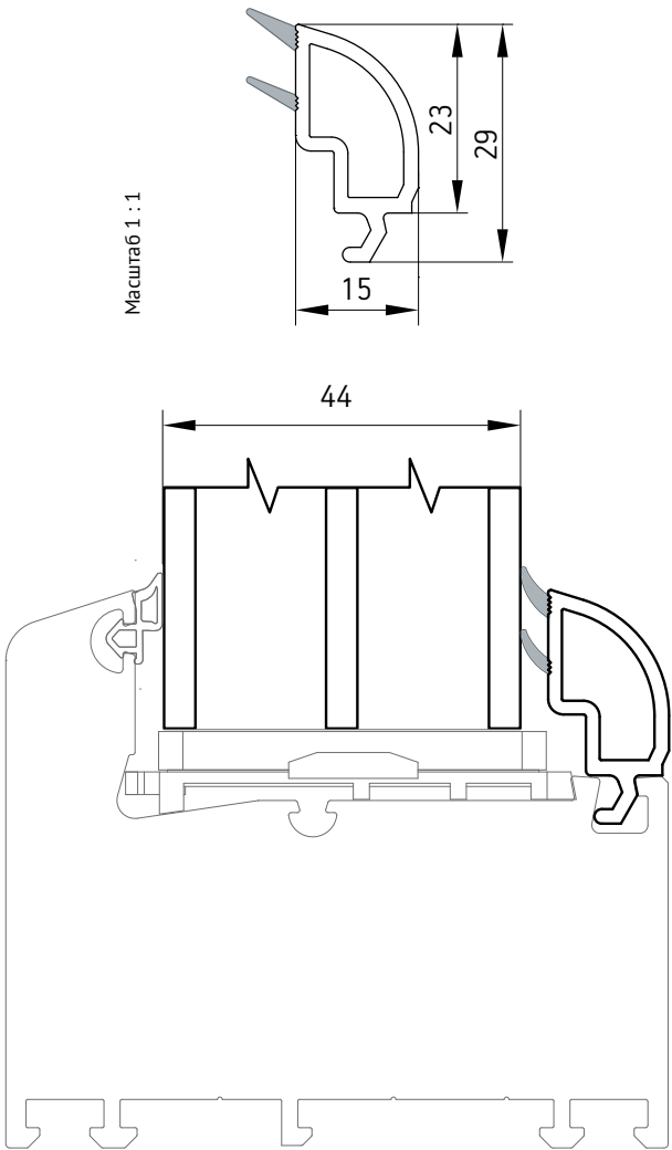
049 Штапик (под стеклопакет 44 мм)
