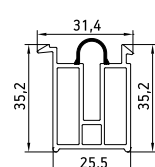
Угловой соединитель 90 023
