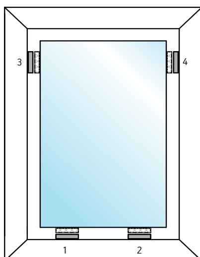
— Фальцевый вкладыш — Дистанционные и несущие подкладки
