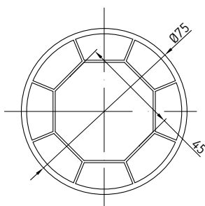
024 Н-соединитель рамы
