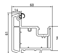
Штульп 60мм 012
