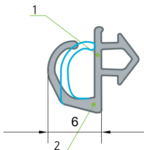
Уплотнитель створки
