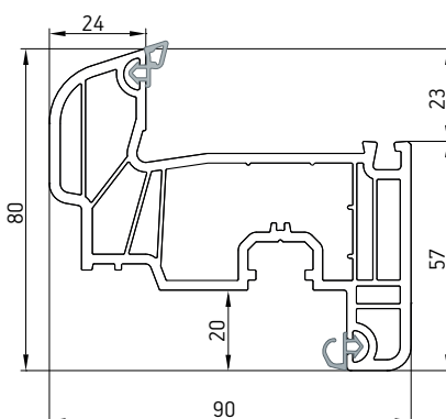
047 Створка 5-камерная
