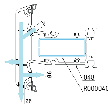
Горизонтальный импост
