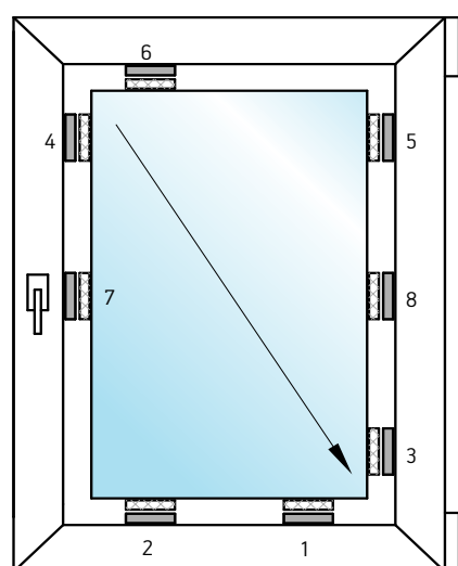
— Фальцевый вкладыш — Дистанционные и несущие подкладки
