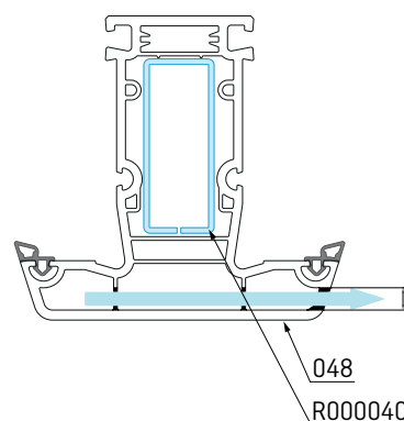
Вертикальный импост
