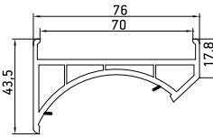
Адаптер кругового коннектора 70 053
