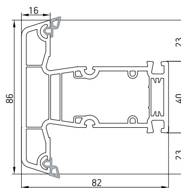
048 Импорт 5-камерный
