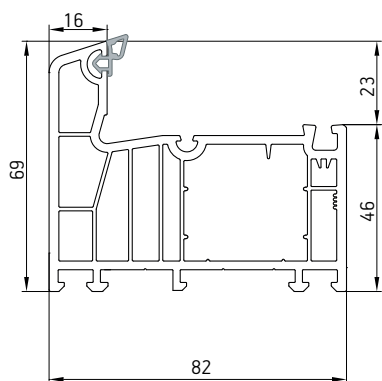
046 Рама 6-камерная
